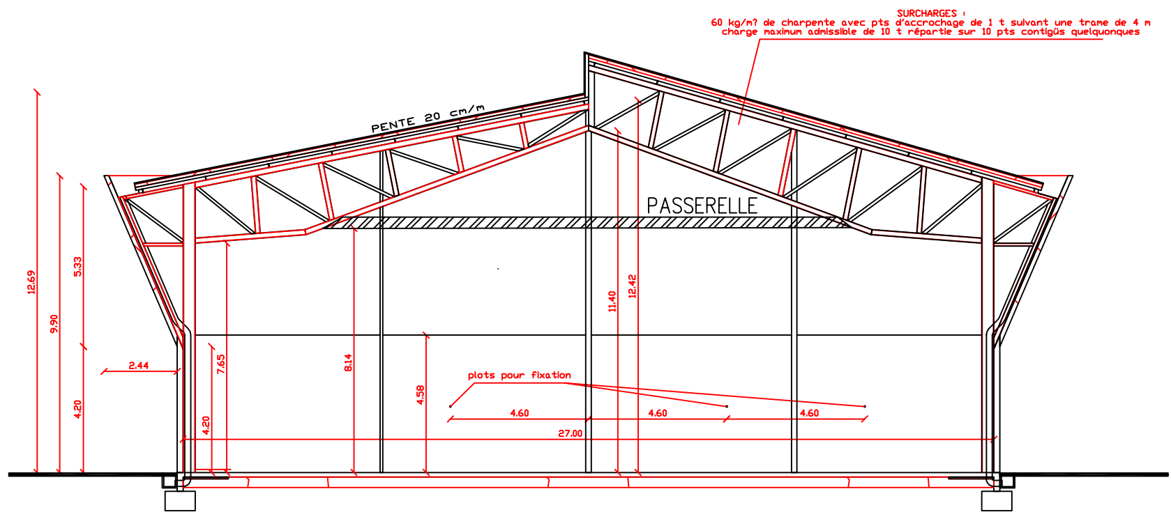
COUPE AA
