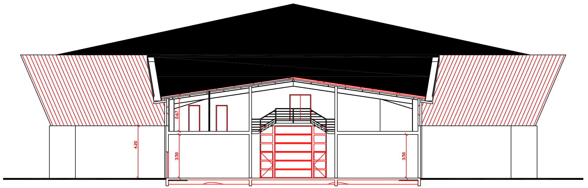
COUPE BB
